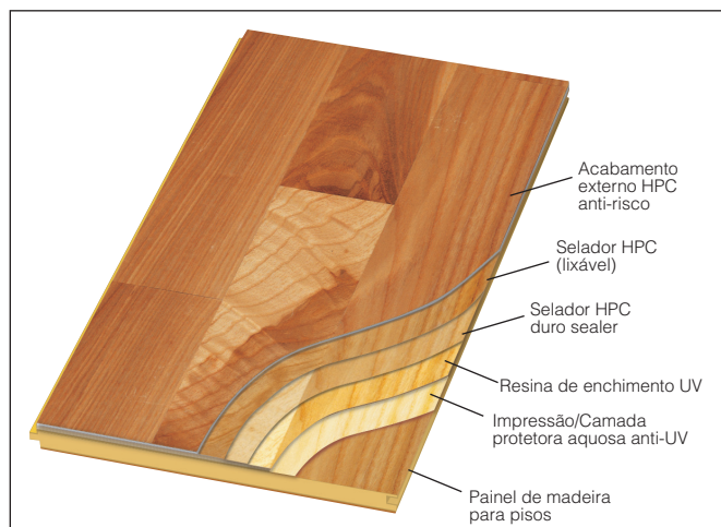
Camadas típicas de pisos de madeira
